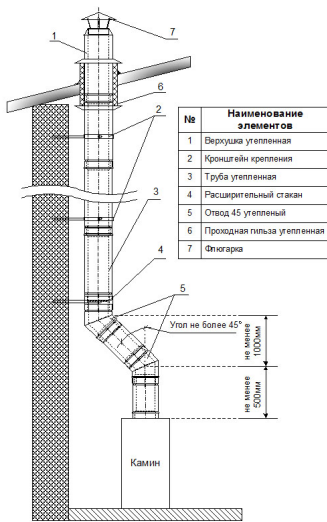
Рис. 8 Типовая конструкция внутреннего утепленного дымохода для камина
