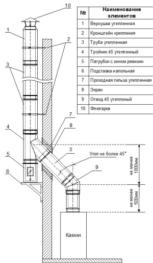
Рис. 7 Типовая конструкция наружного утепленного дымохода для камина
