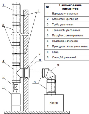
Рис. 6 Типовая конструкция наружного утепленного дымохода для промышленного или бытового котла
